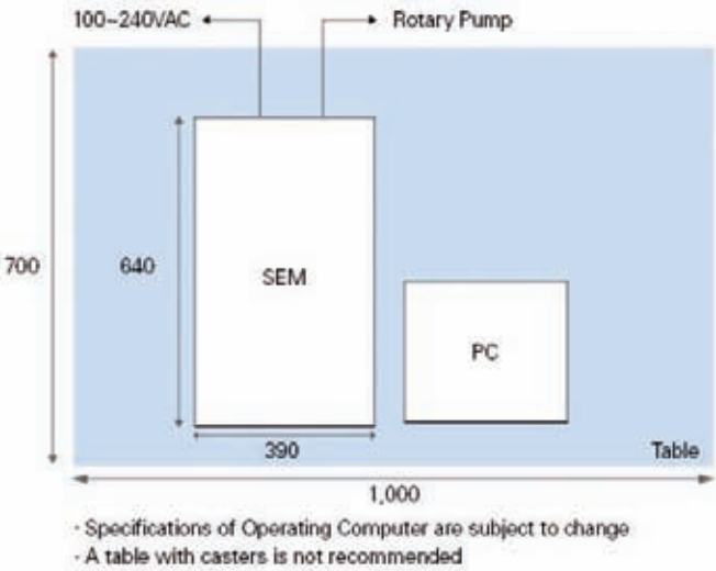
Ejemplo de instalación del escáner MiniSEM
