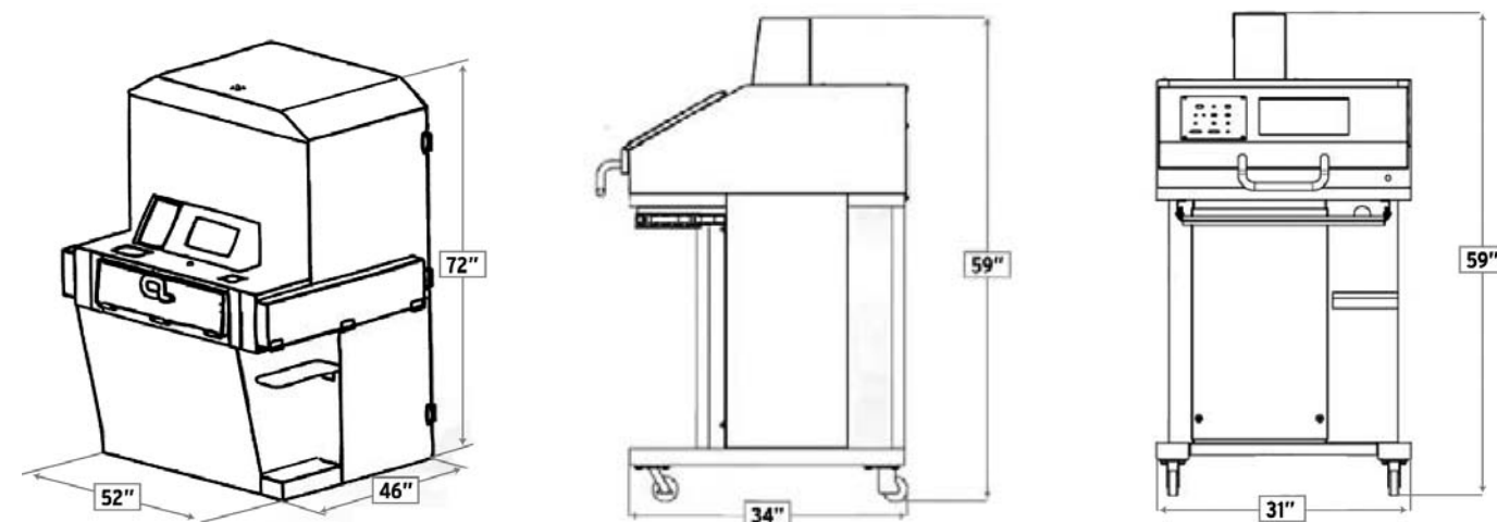
Dimensiones en pulgadas para FSX080-FSX090
